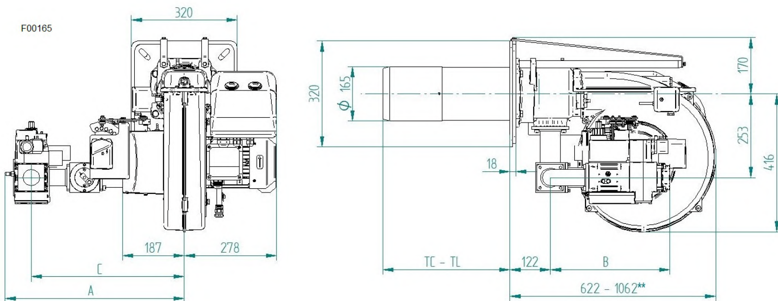
Fig. 3 Dimensions
