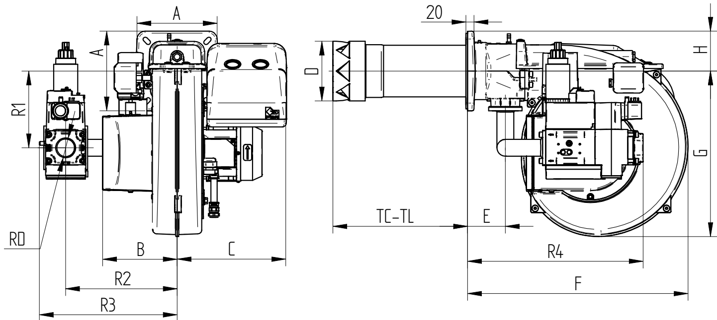
Fig. 2 РАЗМЕРЫ
