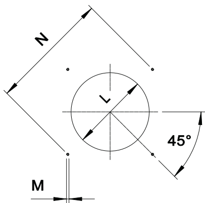
Fig. 3 Фланец для установки горелки
