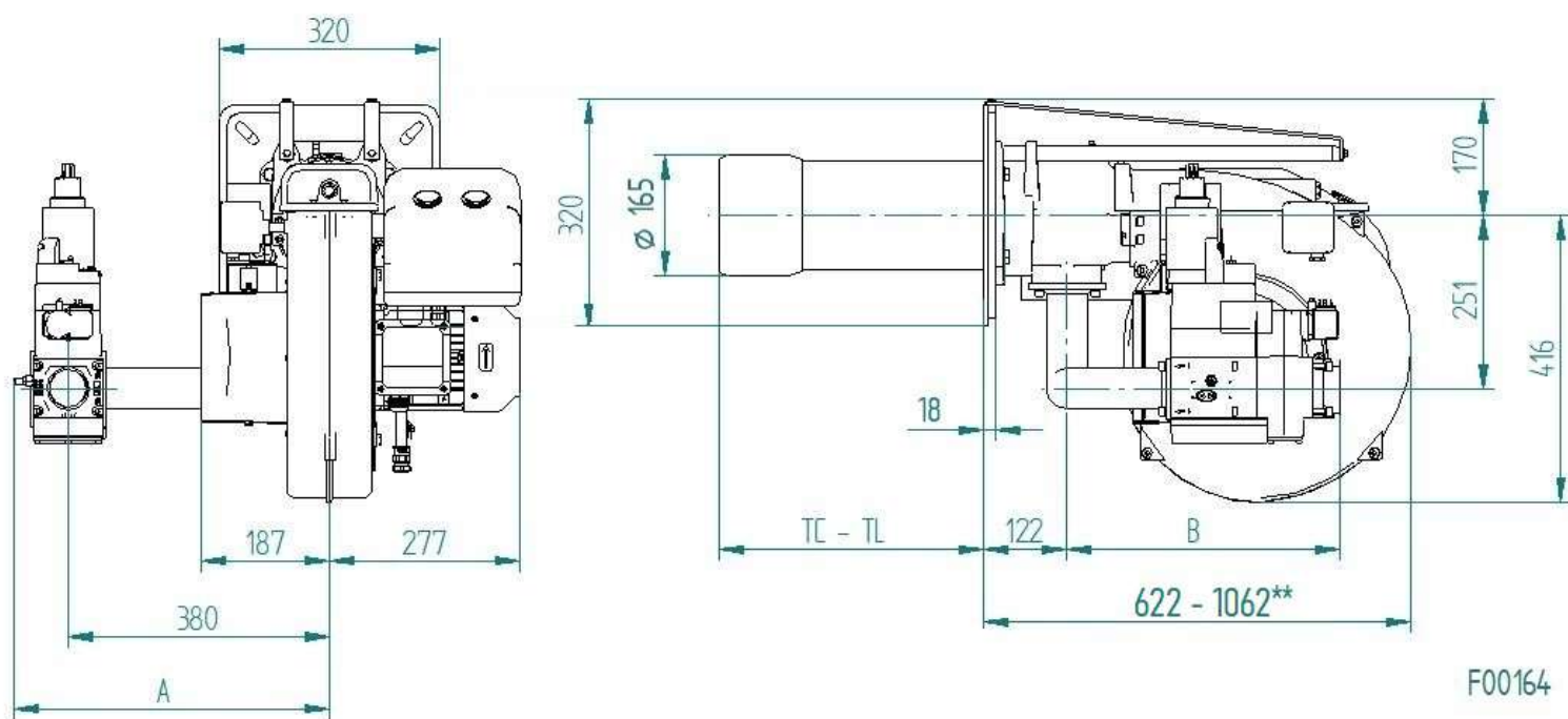
Fig. 3 Dimensions
