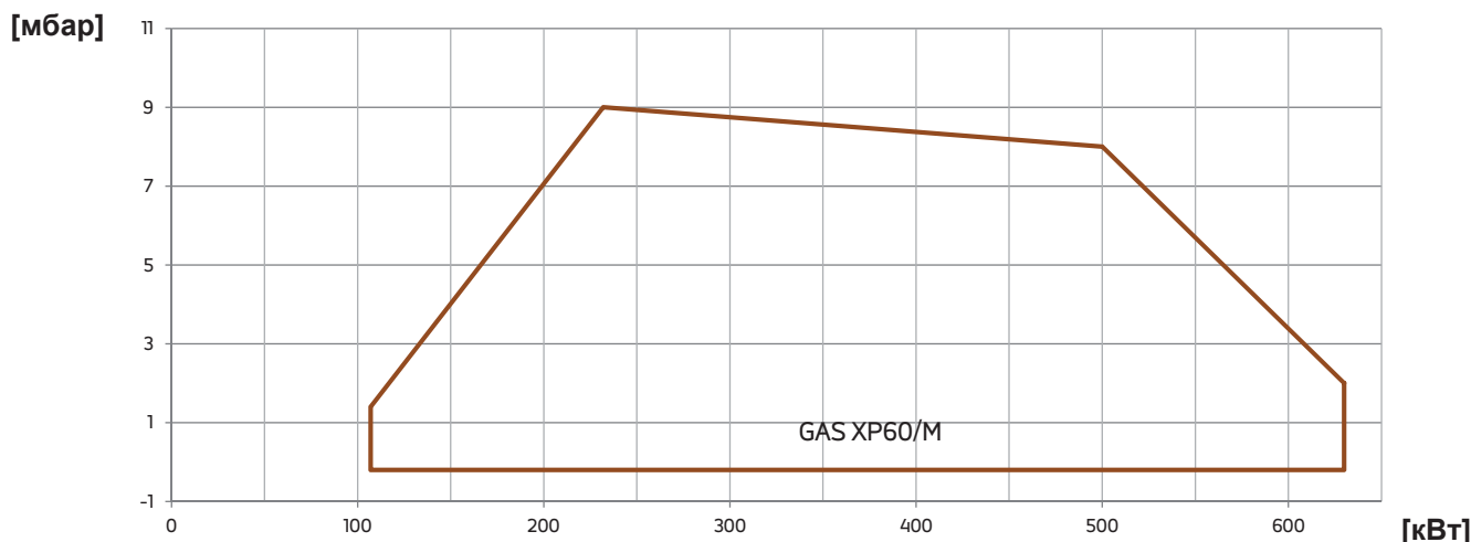
Fig. 2 X = Мощность Y = Соппротивление камеры сгорания
