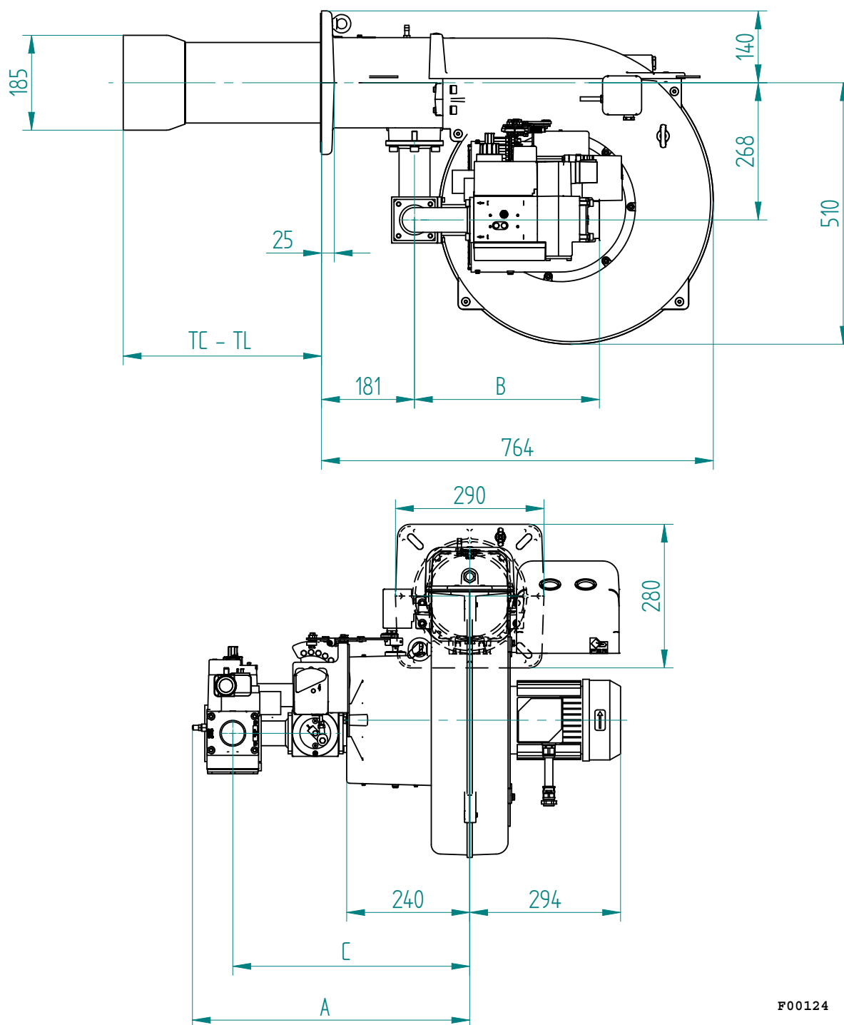
Fig. 3 Dimensions
