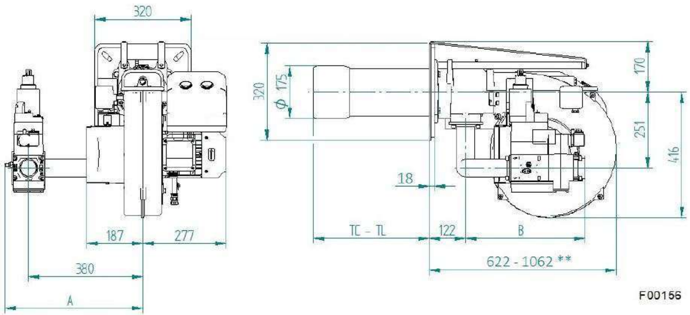
Fig. 3 Dimensions
