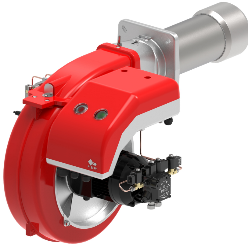
Fig. 1 FGP 50/2 EVO-3
