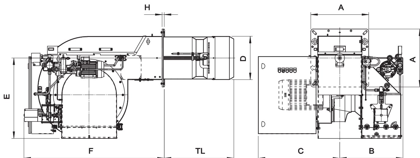
Fig. 3 Burner dimensions
